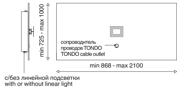
без ниши под кронштейн without a niche for TV holder
