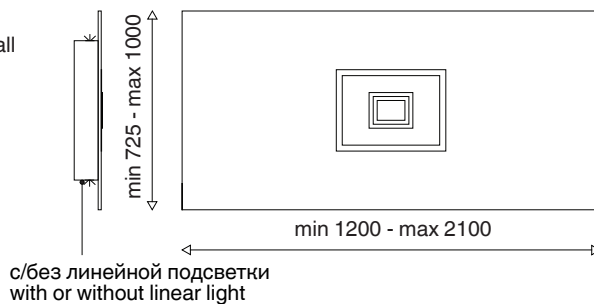
с нишей под кронштейн with a niche for TV holder
