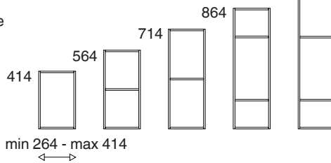
бокс с фасадом | box with door
